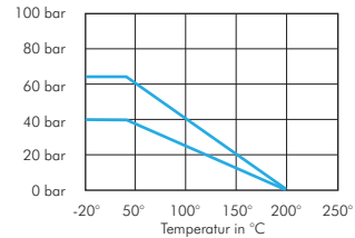
Diagramm 3 - PN 63
