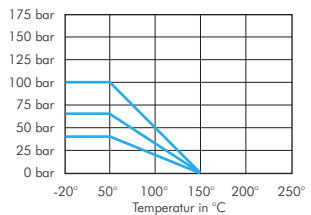
Diagramm 5 - PN 100
